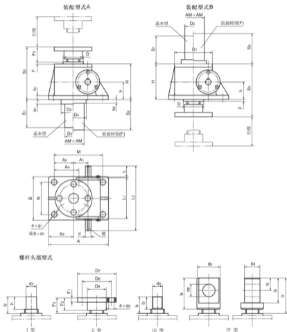
图1 1型结构形式
