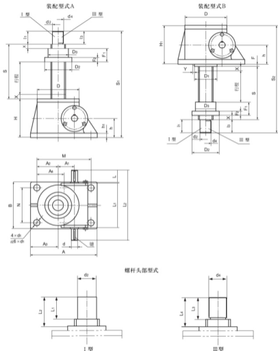
图2 2型结构型式
